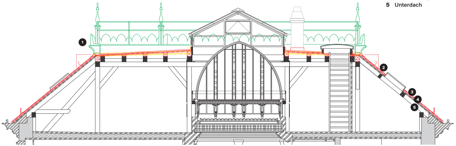
Querschnitt: Die alten Faserzementplatten und die Holzlattung wurde entfernt. Der Dachkranz konnte trotz separater Planung realisiert werden.
