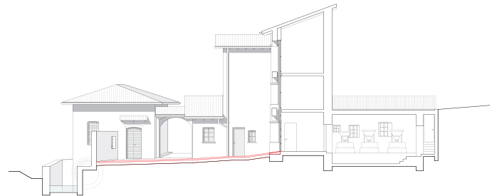
Schnitt. Coupe.
